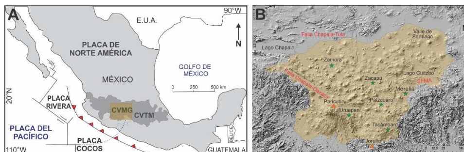
Figura 1. A, Contexto tectónico del Cinturón Volcánico Trans-Mexicano (CVTM) y localización del Campo Volcánico Michoacán-Guanajuato (CVMG). B, Los volcanes Parícutín y Jorullo dentro del Campo Volcánico Michoacán-Guanajuato (área anaranjada), las principales ciudades y estructuras tectónicas. SFMA, Sistema de Fallas Morelia-Acambay.
