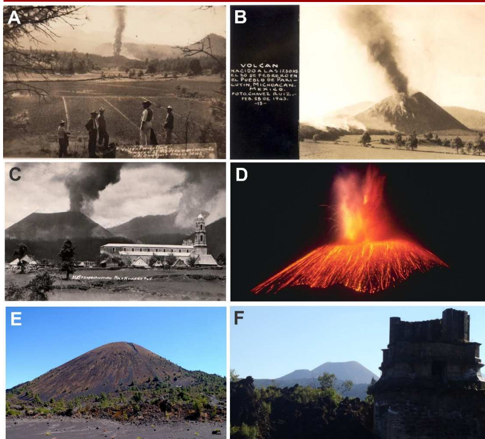
Figura 3. A, Fotografía del Parícutín tomada por Chávez Ruíz el segundo día de su nacimiento. B, Fotografía del crecimiento del volcán, tomada el 28 de febrero de 1943 por Chávez Ruíz. C, Fotografía de la iglesia y pueblo de San Juan Parangaricutiro por Navarro. D, Espectáculo nocturno del volcán Parícutín en erupción, fotografía tomada por Wilcox en 1943. E y F, Apariencia actual del volcán Parícutín y parte de las ruinas de la iglesia en el viejo San Juan Parangaricutiro (Fotografías tomadas por Gómez-Vasconcelos MG en 2017).
